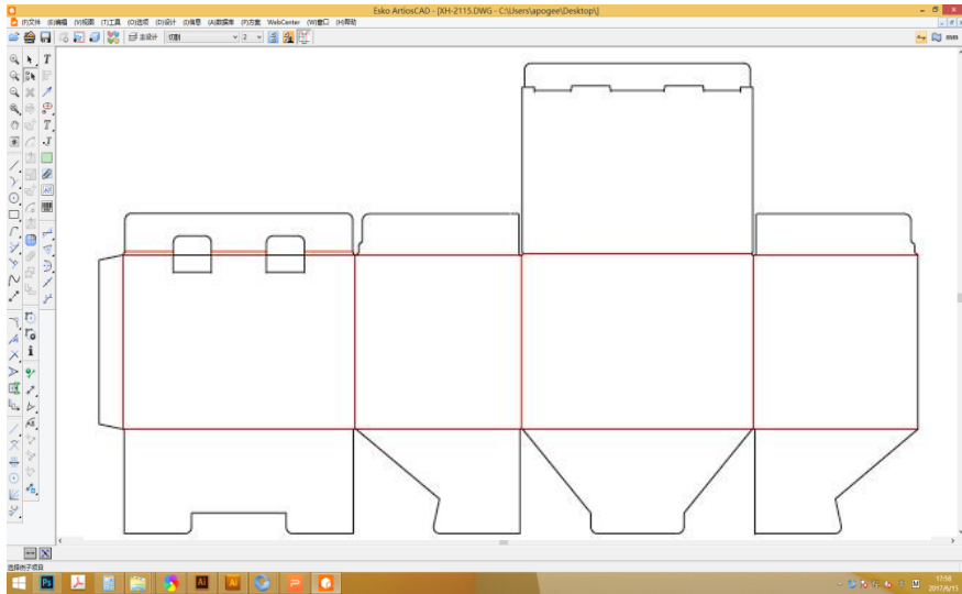
CAD 结构图
